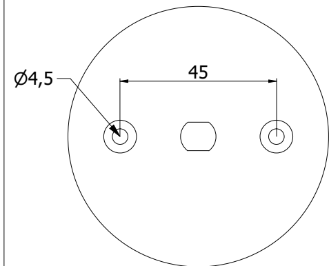
ROZSTAW OTWORÓW MONTAŻOWYCH OPRAWY / MOUNTING HOLES SPACING
